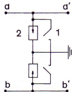
Схема защиты линии разрядником с плавким кольцом
